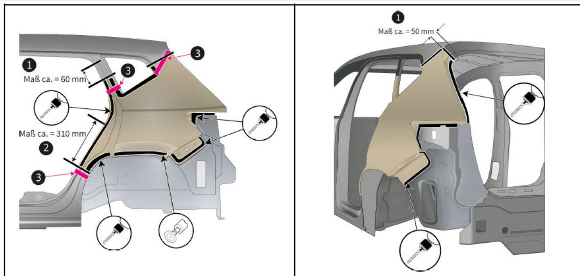
Bild 1: Seitenteil Ausbau
